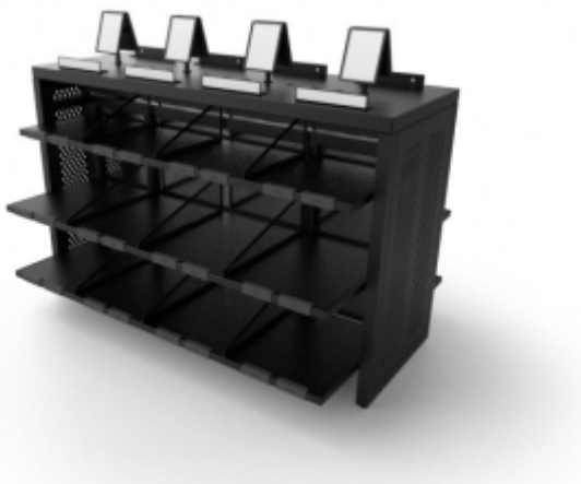
PSF82.2 - BOTTON BAR TABLE A: 1440 B: 1000 H: 750
